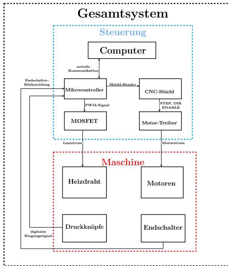
Abbildung 17.1.: Schematische Darstellung des CNC-Heißdrahtschneiders als Automatisierungssystem
