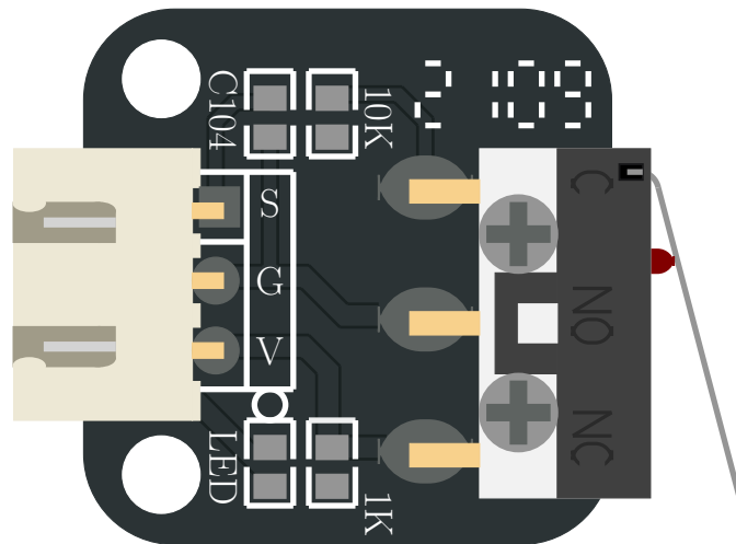
Abbildung 11.1.: Darstellung des im Projekt verwendeten Endschalters
