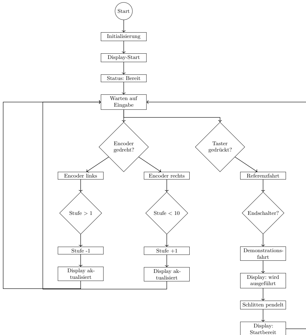
Abbildung 15.4.: Flussdiagramm des Programms
